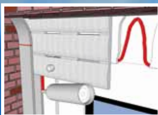
Verklebung und Abdichtung im Bereich der Rolladenführungsschienen
