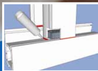
Abdichtung im Bereich der Kämpfer-T-Verbindung
