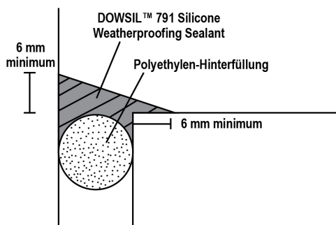
Abbildung 3: Dreiecksfuge
