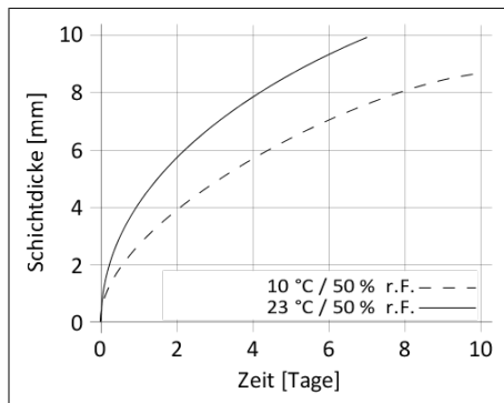
Diagramm 1: Durchhärtengeschwindigkeit Sikaflex®-221i
